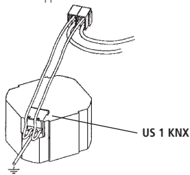
Bild 1: Anordnung des US 1 KNX direkt am Busankoppler
