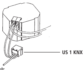
Bild 2: Anschluß des US 1 KNX an der vorhandenen Busklemme des Busankopplers
