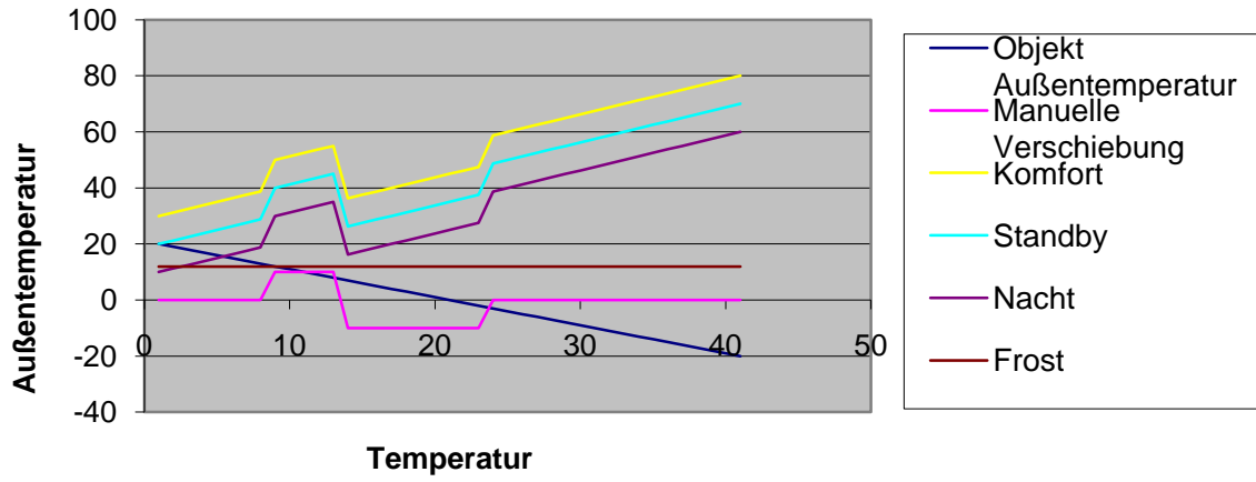
Abbildung 6: Vorlaufsollwert in Abhängigkeit der Außentemperatur bei den verschiedenen HKL Betriebsarten.
